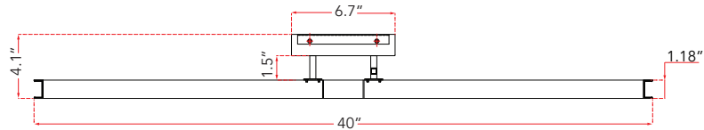
Top Elevation
